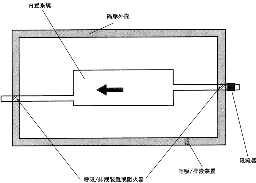
图 G.1 具有内置系统的隔爆外壳
