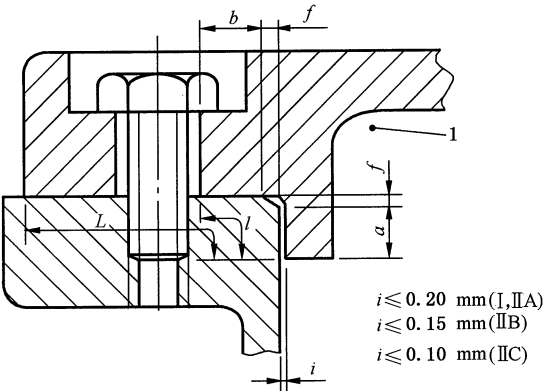
图4 平面接合面上的孔(示例2)
